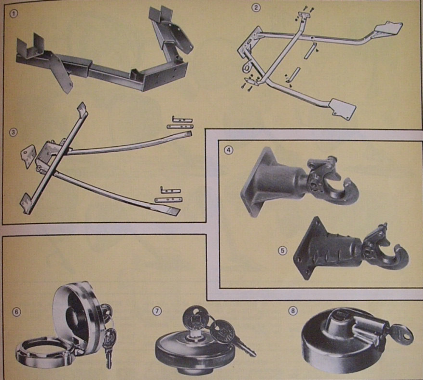
① DISPOSITIF d'attelage de remorque. (Pour montage, voir N.T. n° 254.)
